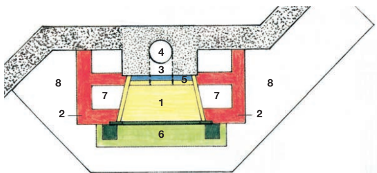
Figura 4. Planul de bază realizat pentru meșterul sobar
